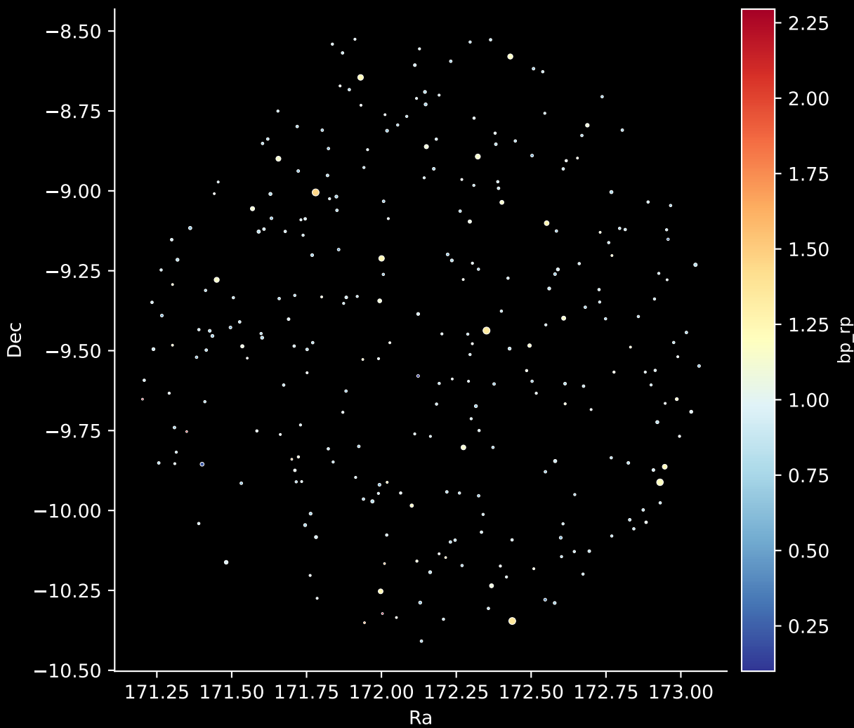
GALAH DR4 Field: [841] Stars: 284
