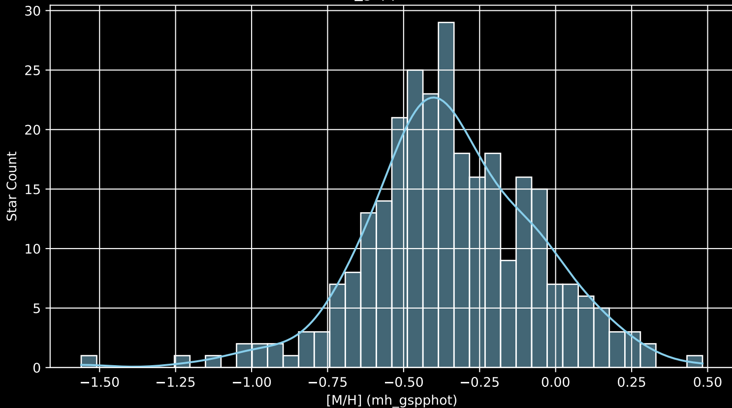
GALAH DR4 Field: [841] [M/H] (mh_gspphot) (n= 282)
