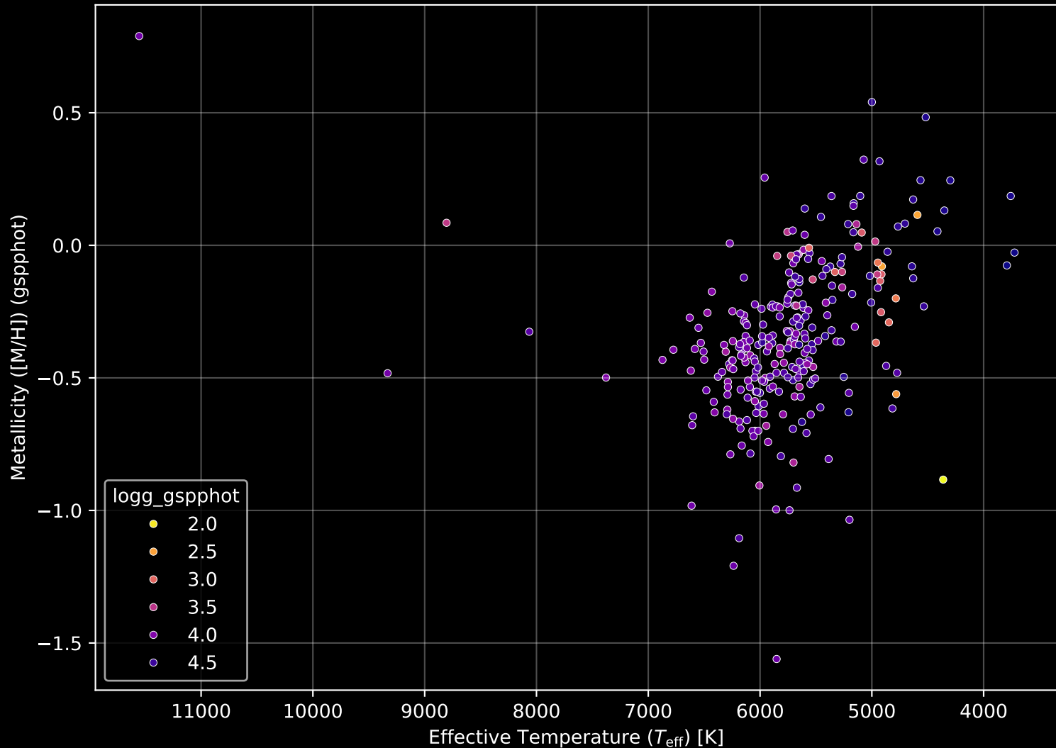
GALAH DR4 Field: [841] Stellar Population Parameters (n= 284)
