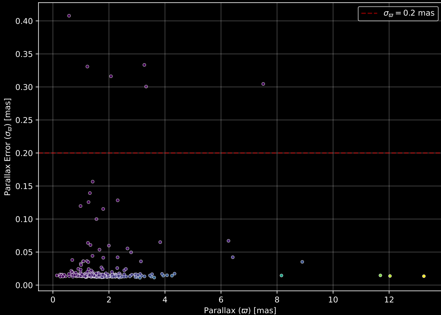
GALAH DR4 Field: [841] Parallax Quality (n= 284)
